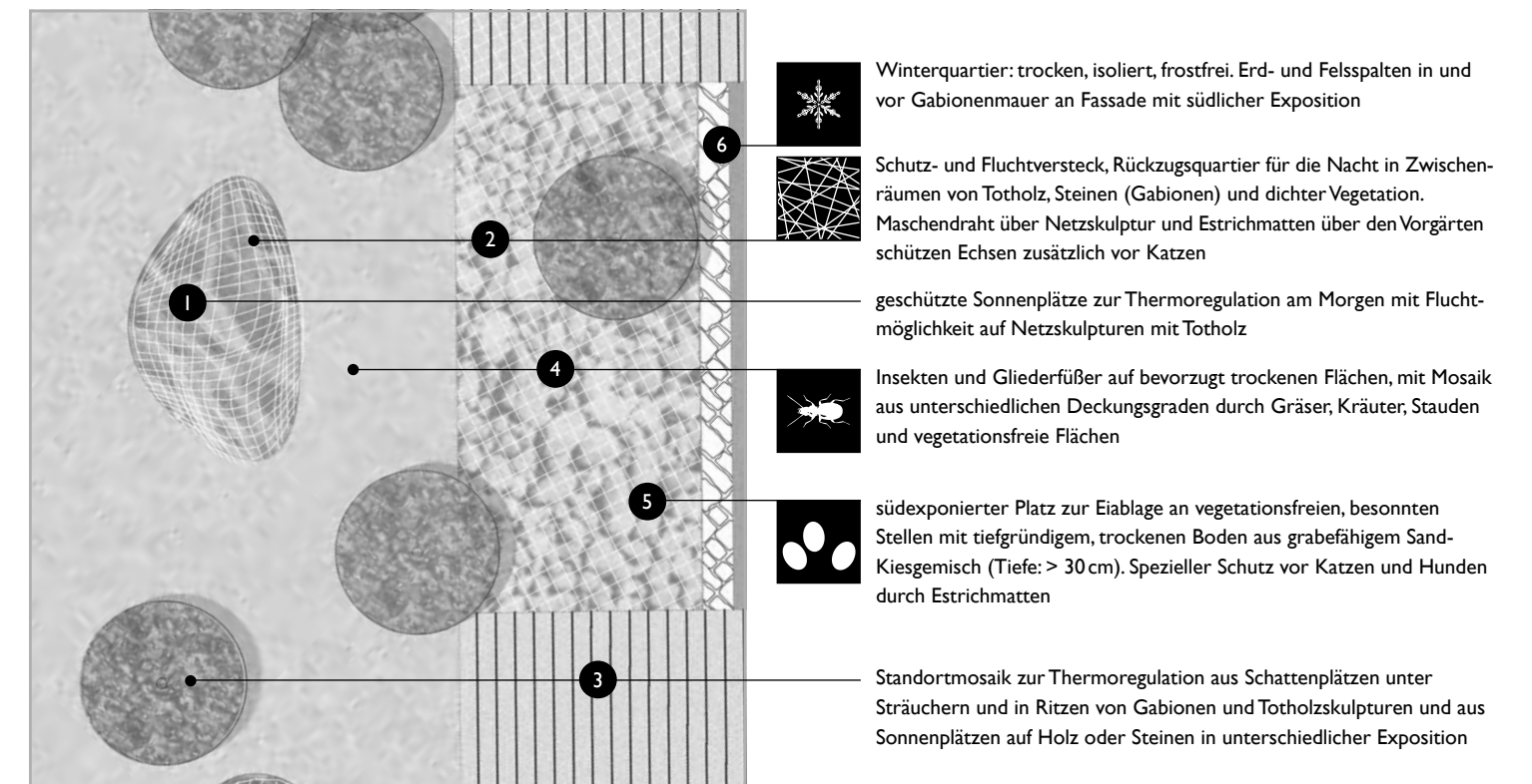
Ausschnitt Lageplan
