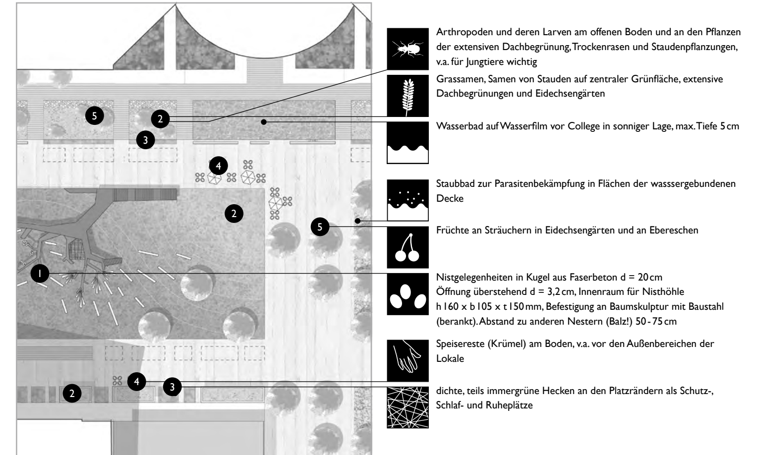
Ausschnitt Lageplan
