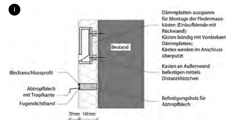
Schnitt Fassadenquartier: Quelle: Architekturbüro Hechenbichler, München
